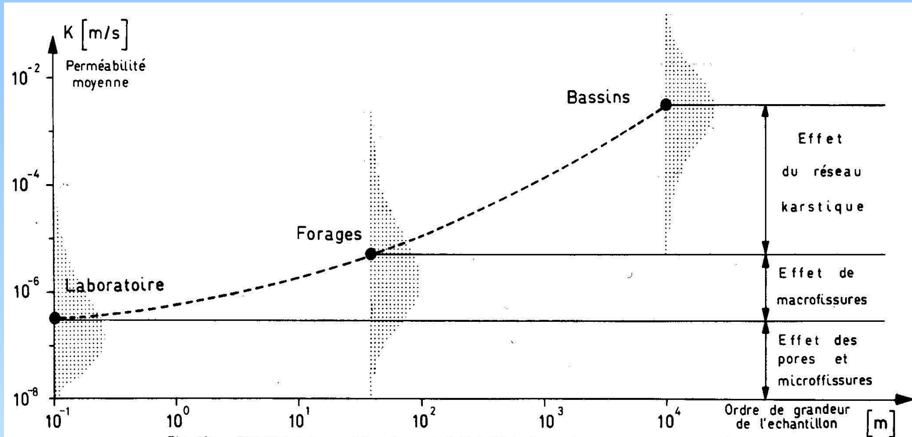
Fig. 19. — Représentation schématique de l'effet d'échelle sur la perméabilité dans le karst.
